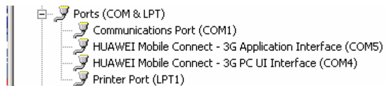
Abbildung 1: Windows Gerätemanager
